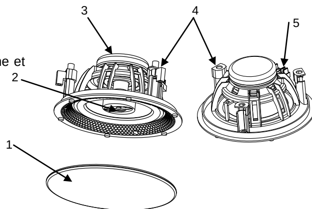
Figure 1. Haut-parleur LS3
