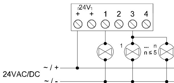
Figure 2: Exemple de connexion: une vanne par sortie et plusieurs vannes par sortie.
