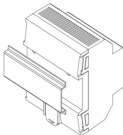
Figure 3. Montage du NarrowDIM X4 sur rail DIN
