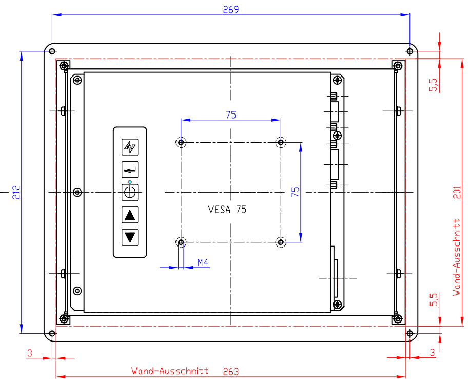
RÜCKANSICHT
