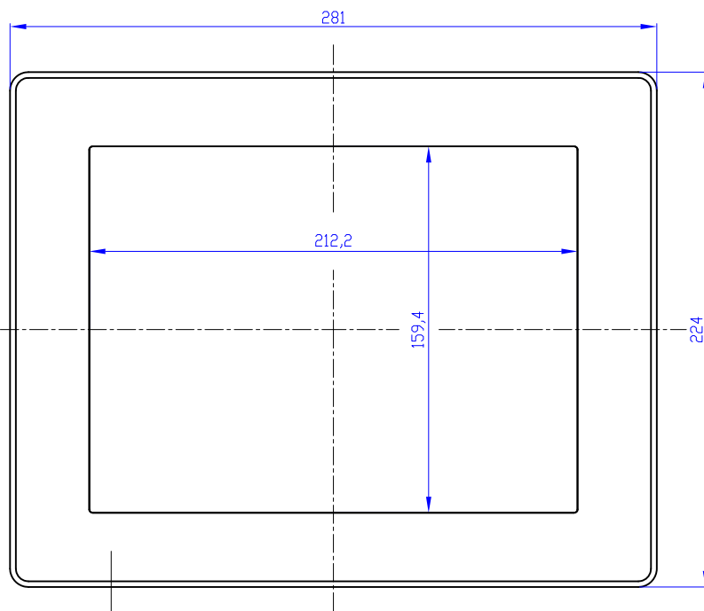
FRONTANSICHT
