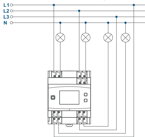
Raccordement de différentes charges (sorties) :
