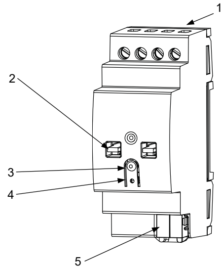
Abbildung 1: IndustrialBOX Current 2
